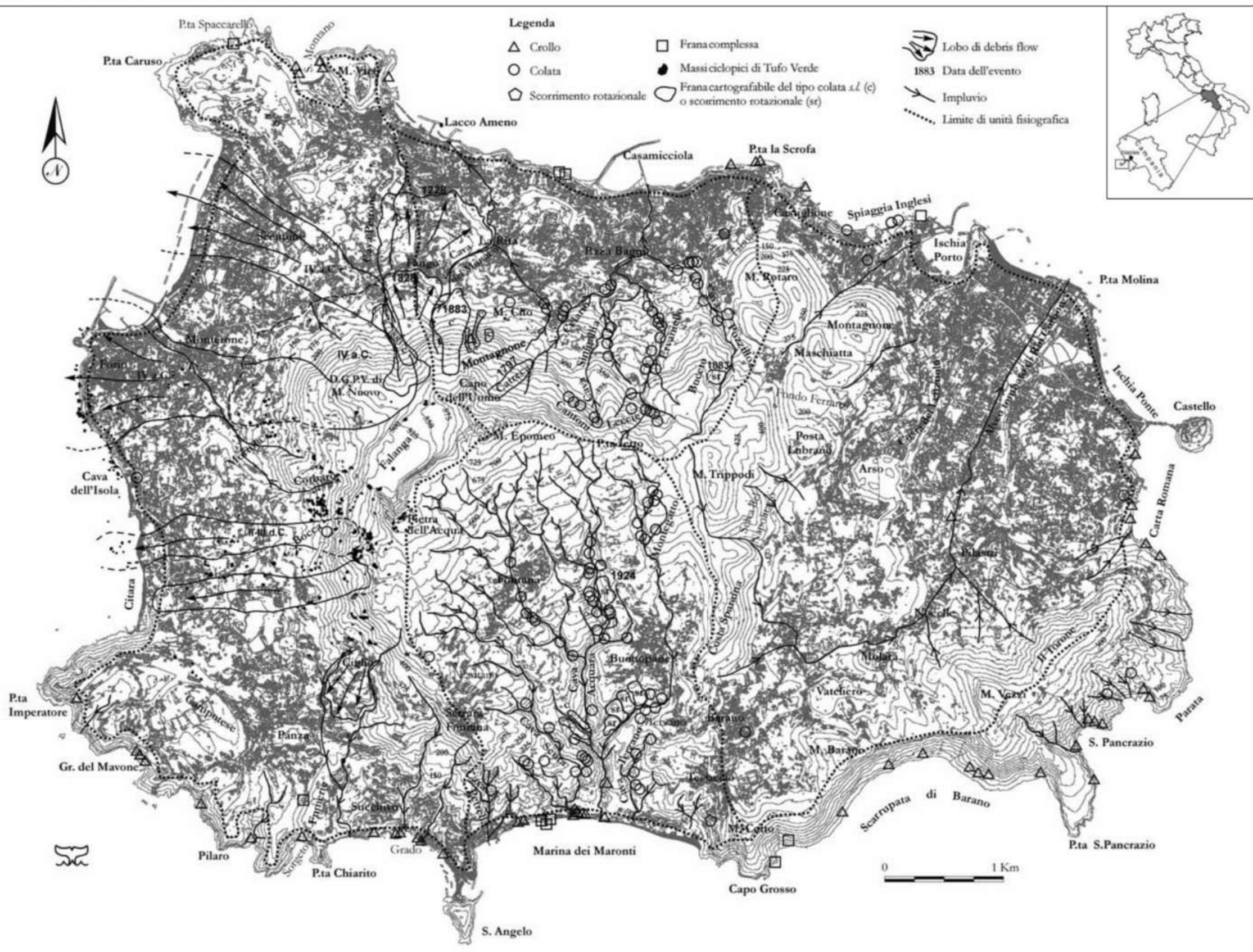
Fig. 2 - Carta degli ambiti fisiografici e delle frane dell'isola d'Ischia. Per motivi di leggibilità sono riportate solo le date, qualora note, degli eventi franosi cartografabili di maggior rilievo. - Physiographic and landslides map of Ischia island. For better reading of the map we have report only the age, if note, of major landslides event.
