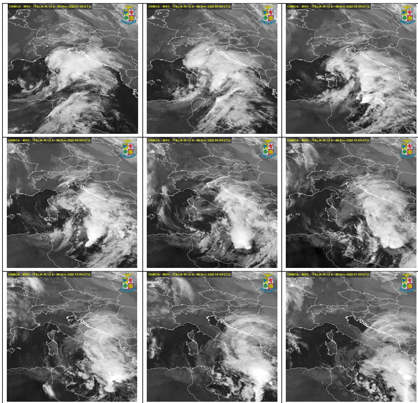
Figura 15 - Sequenza di immagini trionaria del satellite nel canale IR 10.8 dalle ore 21:00 UTC del 25 novembre 2022 alle ore 21:00 UTC del 26 novembre 2022.
