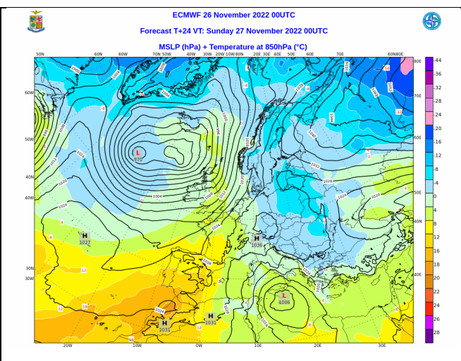
Figura 8: Mapa di previsione della pressione media a livello del mare e temperatura a 850hPa alle 00UTC del 27 novembre 2022(RUN delle 00UTC del 26 novembre 2022).
