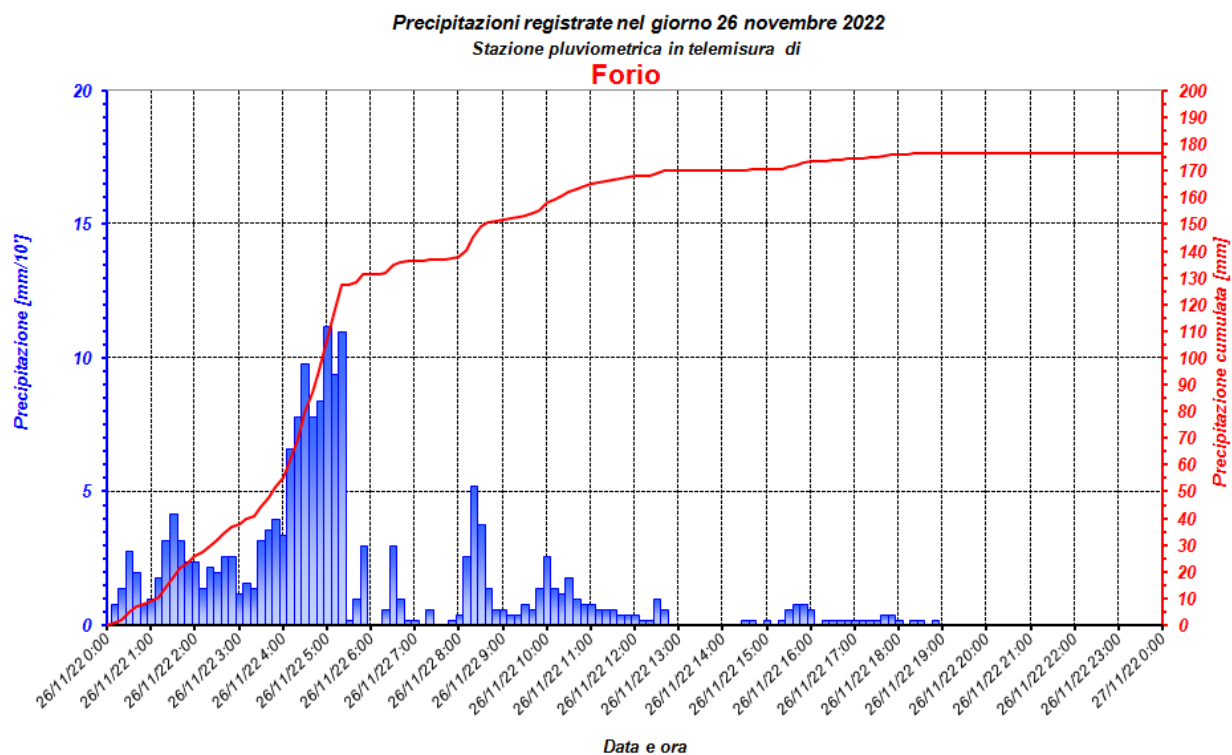
Figura 19 - Pluviogramma delle precipitazioni e relativa precipitazione cumulata. Stazione di Forio.
