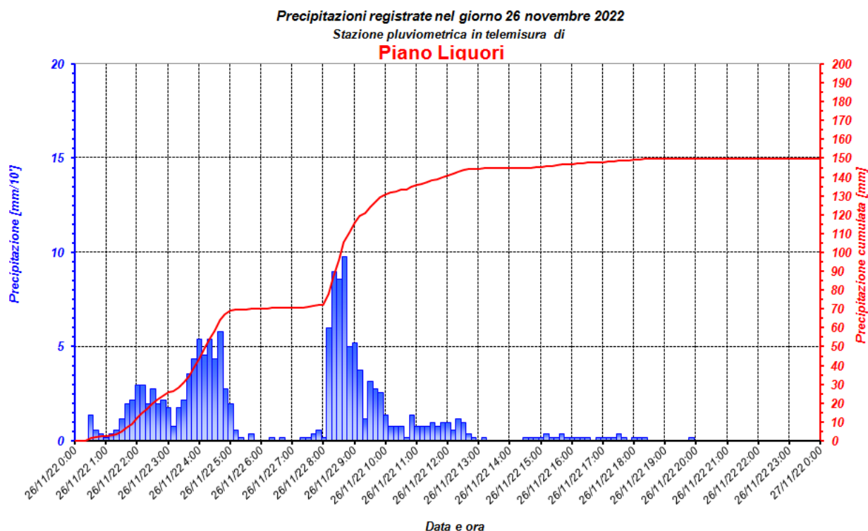
Figura 21 - Pluviogramma delle precipitazioni e relativa precipitazione cumulata. Stazione di Piano Liguori.
