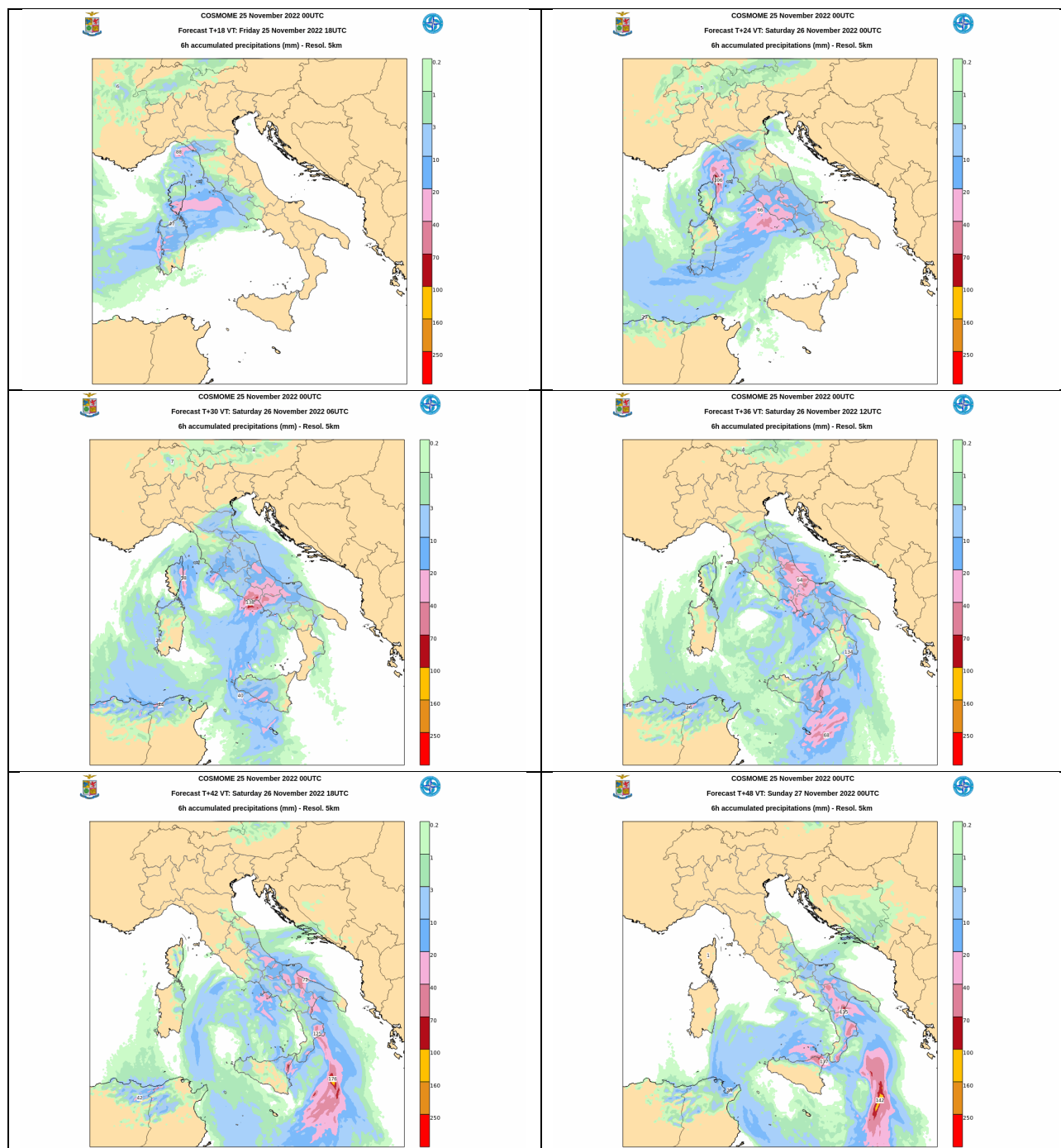
Figure 11 - Mappe di previsione delle precipitazioni cumulate nelle 6 ore precedenti dalle ore 18UTC del 25 novembre 2022 alle 00UTC del 27 novembre 2022 del modello COSMOME (RUN delle 00 UTC del 25 novembre 2022).
