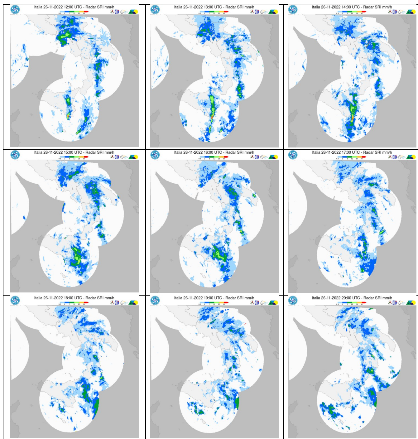
Figura 16 - Sequenza di immagini orarie della mosaicatura RADAR del Dipartimento della Protezione civile dalle ore 21:00 UTC del 25 novembre 2022 alle ore 20:00 UTC del 26 novembre 2022.
