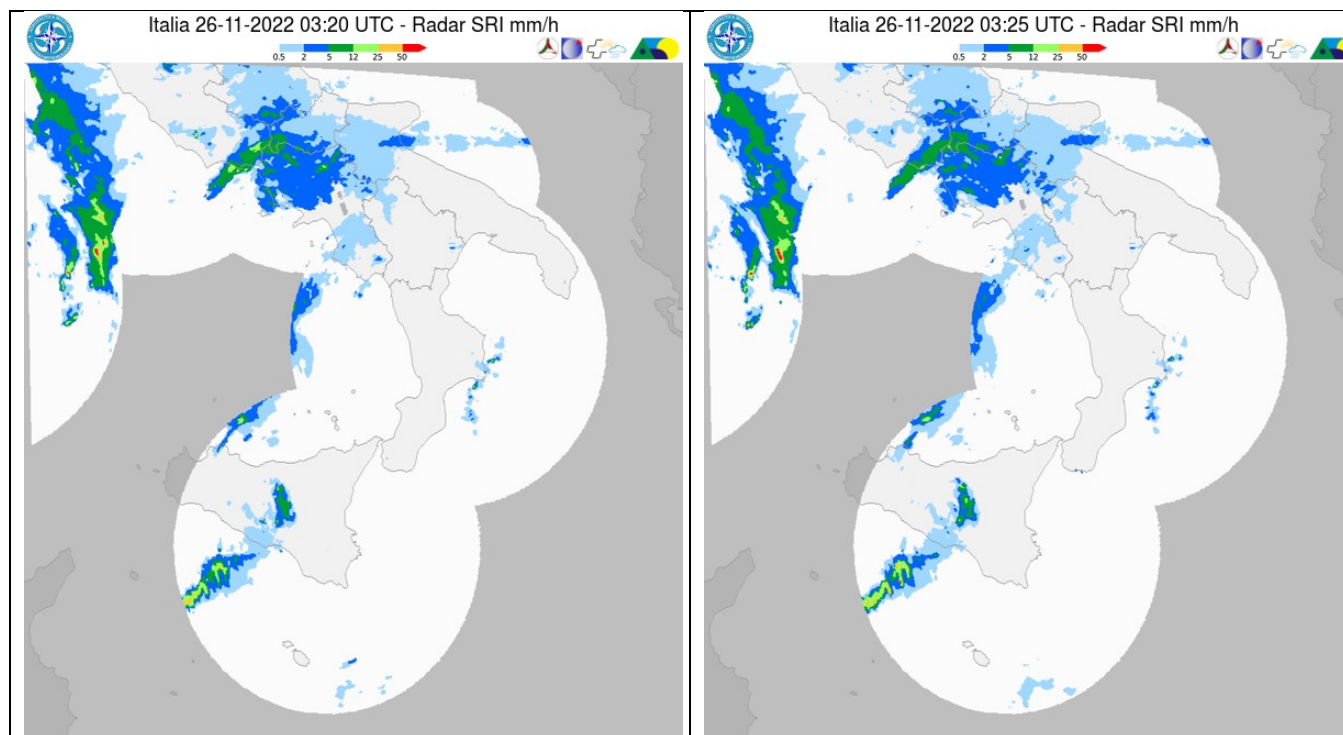
Figura 17 - Sequenza di immagini, con intervallo di rilevazione pari a 5 minuti, della mosaicatura RADAR del Dipartimento della Protezione civile dalle ore 01:00 UTC alle ore 03:25 UTC del 26 novembre 2022.
