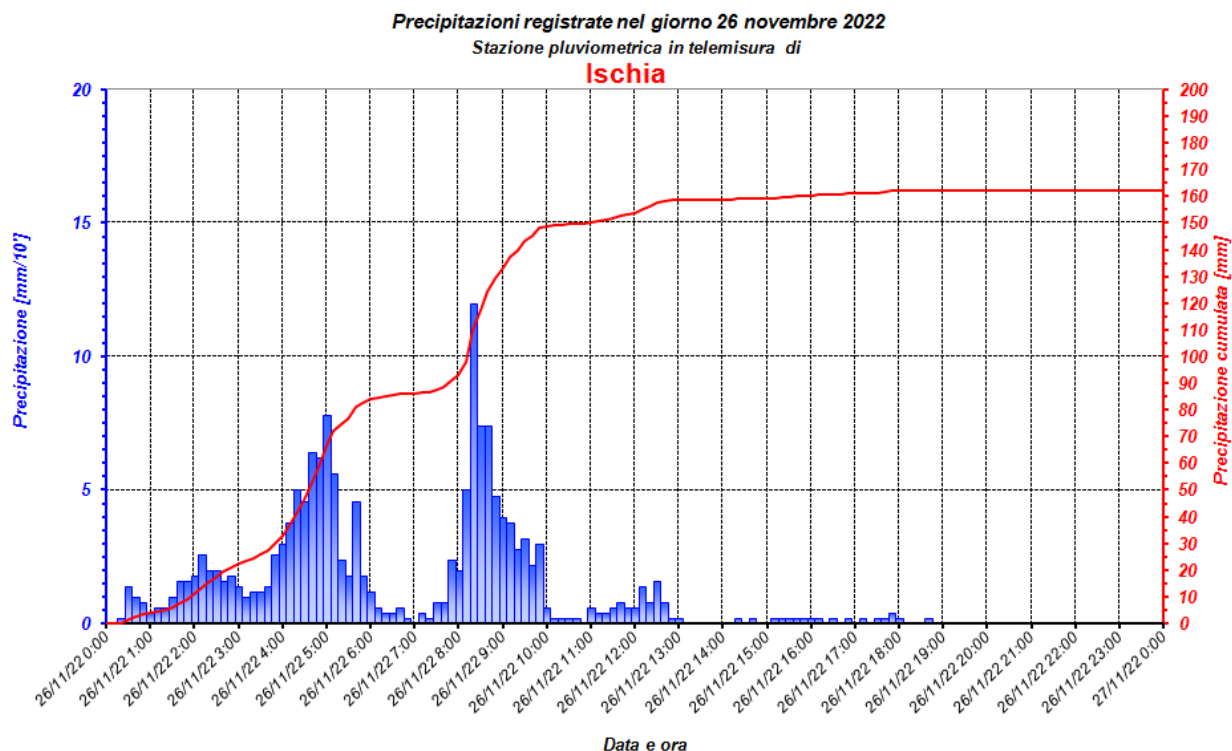
Figura 20 - Pluviogramma delle precipitazioni e relativa precipitazione cumulata. Stazione di Ischia.
