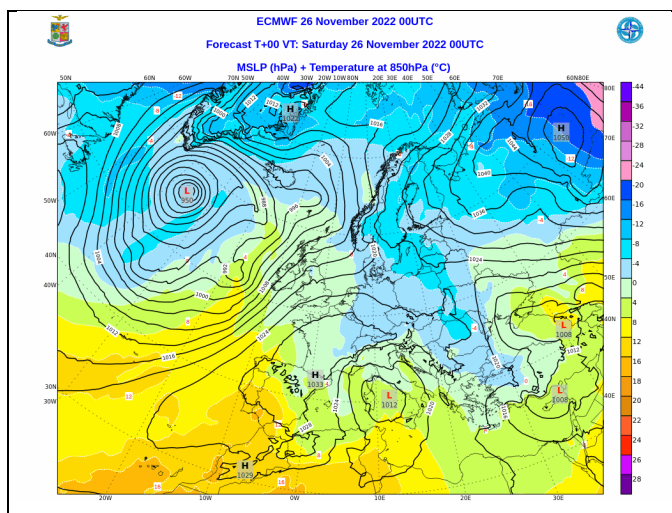
Figura7: Mapa di previsione della pressione media a livello del mare e temperatura a 850hPa alle 00UTC del 26 novembre 2022(RUN delle 00UTC del 26 novembre 2022).
