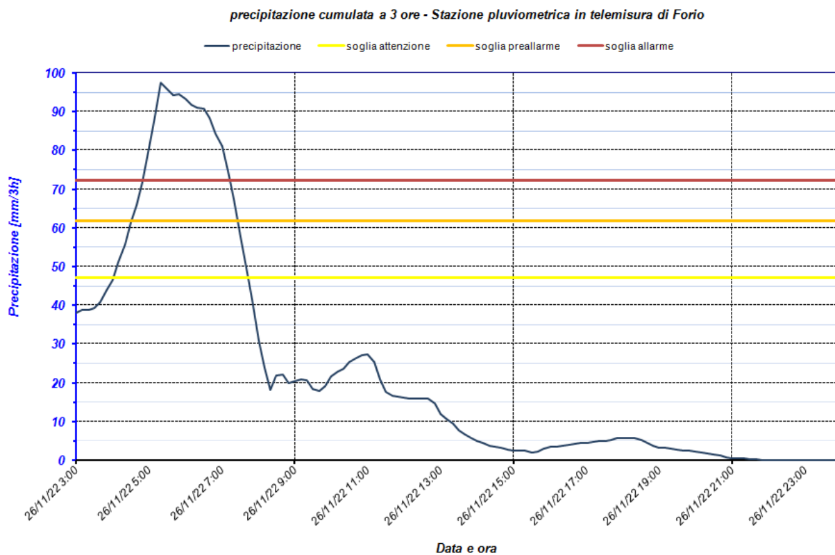
Figura 24. Stazione di Forio: andamento temporale del precursore pluviometrico di durata 3 ore.
