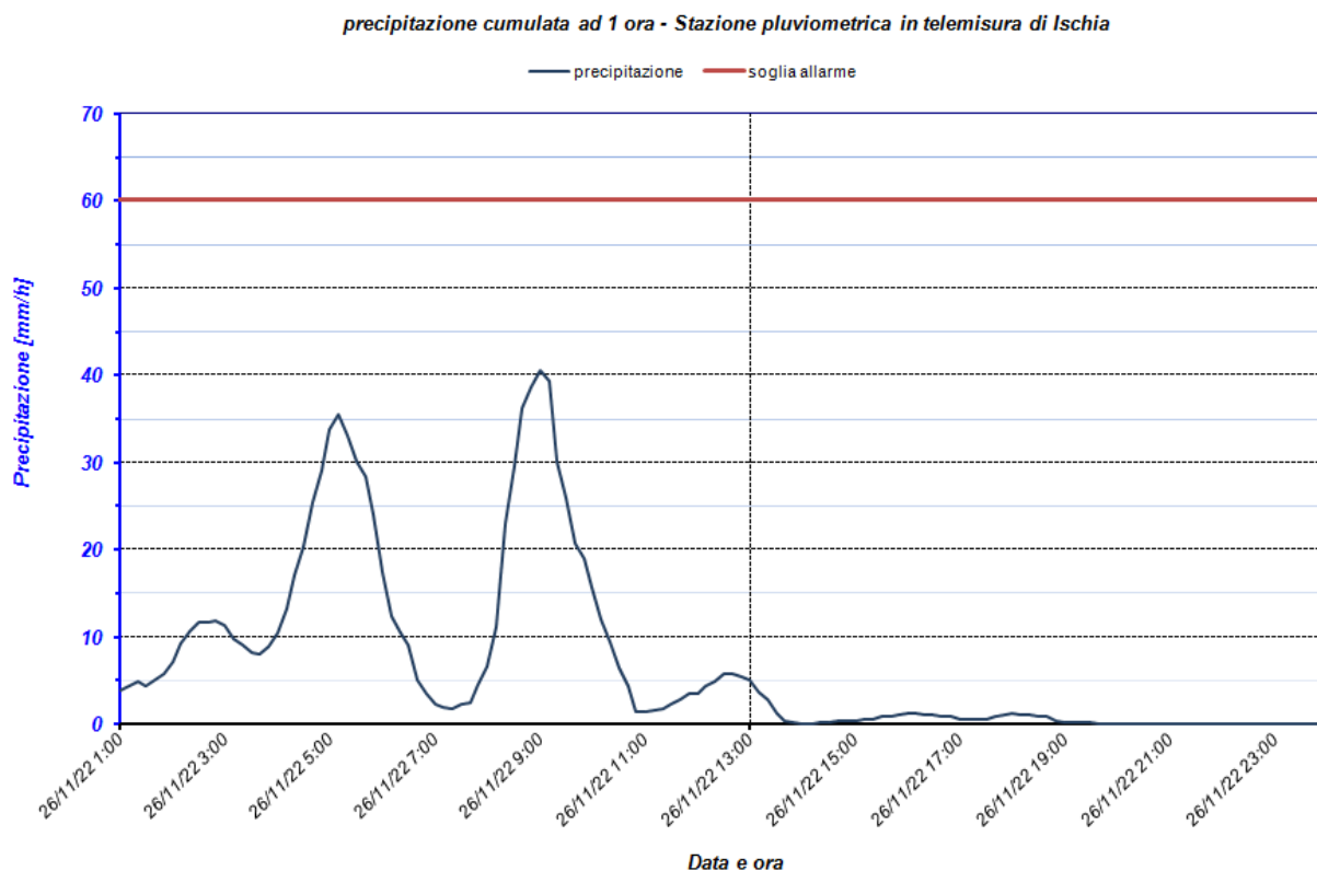
Figura 25. Stazione di Ischia: andamento temporale del precursore pluviometrico di durata 1 ora.
