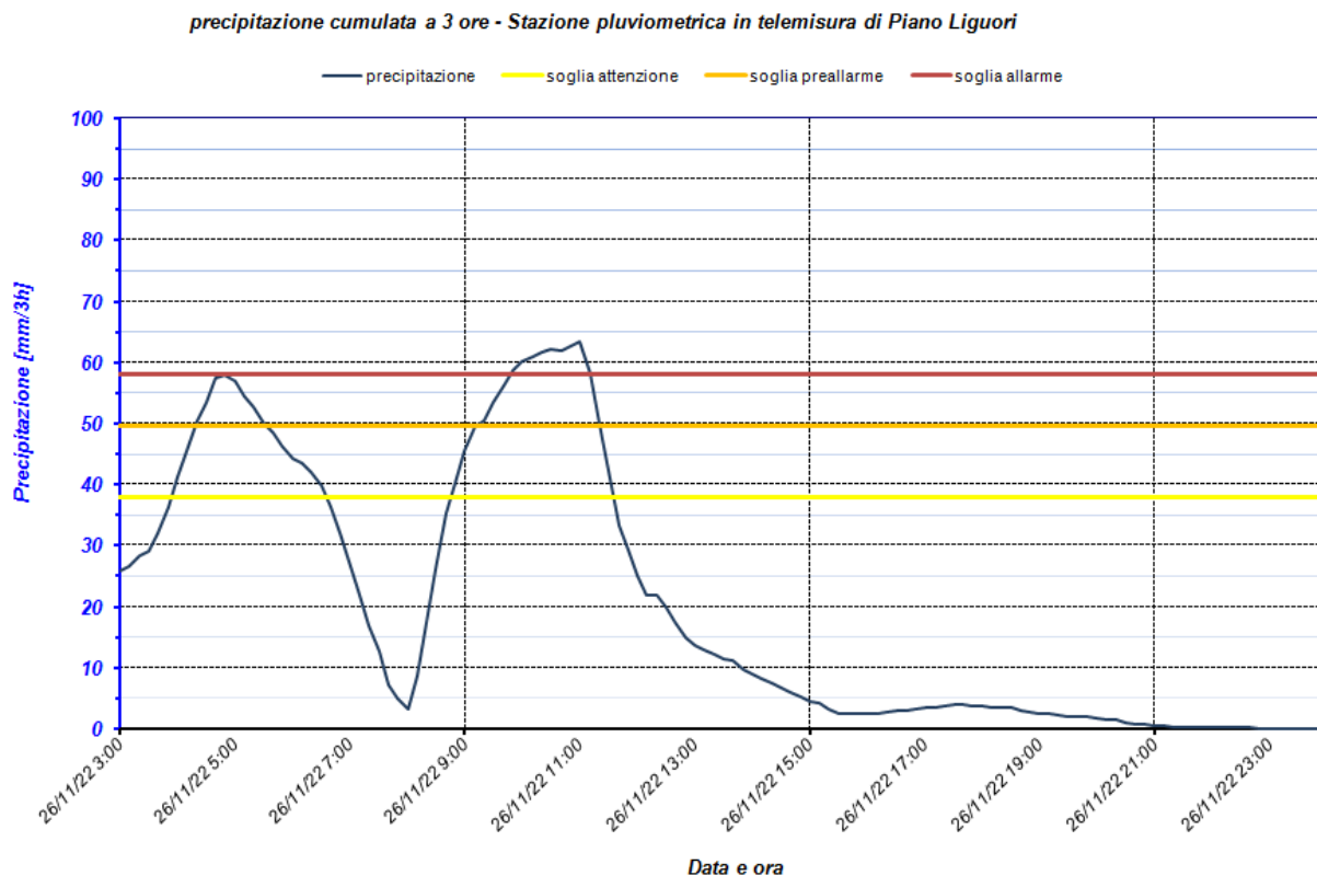
Figura 28. Stazione di Piano Liguori: andamento temporale del precursore pluviometrico di durata 3 ore.
