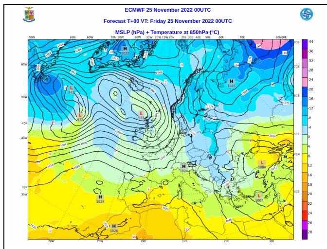
Figura 5: Mapa di previsione della pressione media a livello del mare e temperatura a 850hPa alle 00UTC del 25 novembre 2022 (RUN delle 00UTC del 25 novembre 2022).
