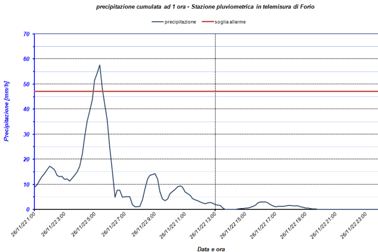
Figura 23. Stazione di Forio: andamento temporale del precursore pluviometrico di durata 1 ora.
