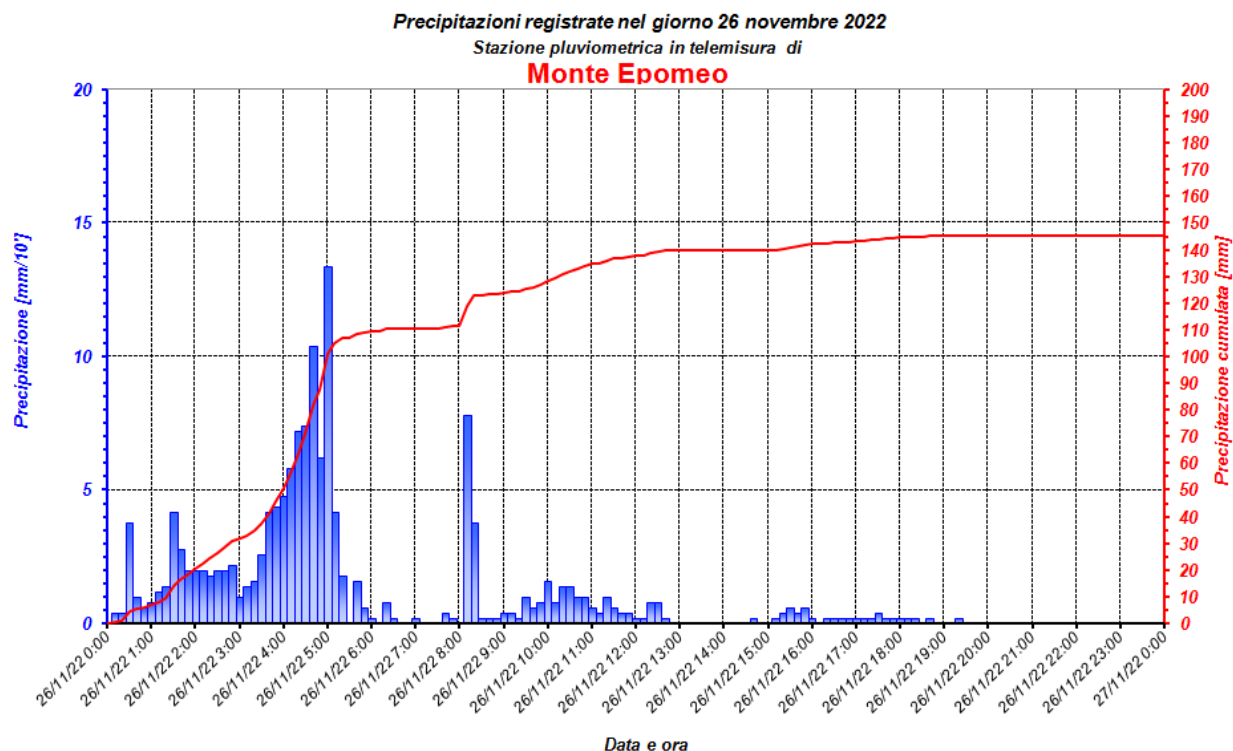
Figura 22 - Pluviogramma delle precipitazioni e relativa precipitazione cumulata. Stazione di Monte Epomeo.
