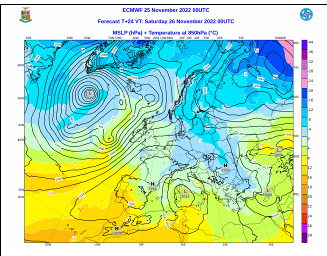
Figura 6: Mapa di previsione della pressione media a livello del mare e temperatura a 850hPa alle 00UTC del 26 novembre 2022 (RUN delle 00UTC del 25 novembre 2022).
