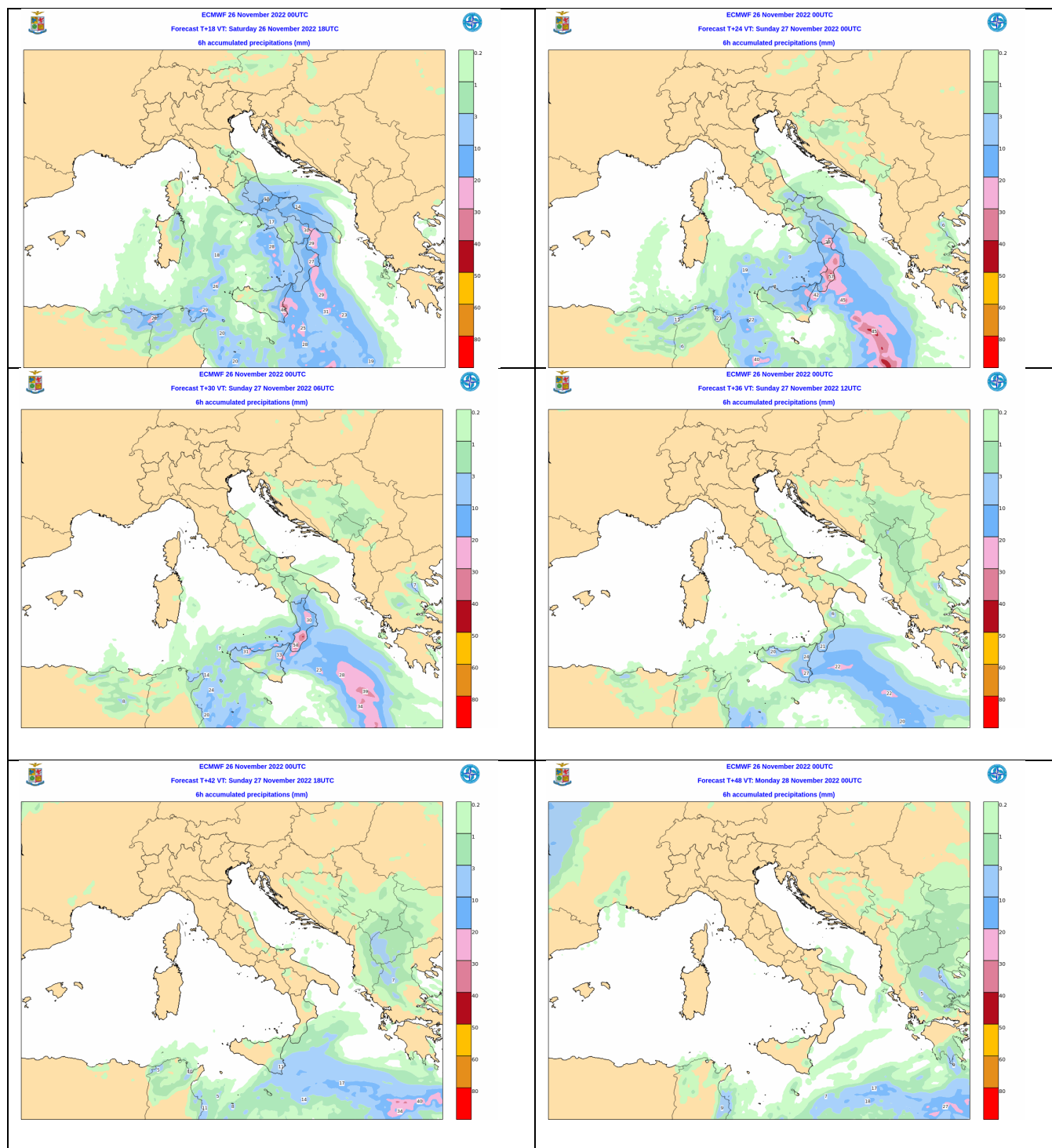
Figure 10 - Mappe di previsione delle precipitazioni cumulate nelle 6 ore precedenti dalle ore 18UTC del 26 novembre 2022 alle 00UTC del 28 novembre 2022 del modello ECMWF (RUN delle 00 UTC del 26 novembre 2022).
