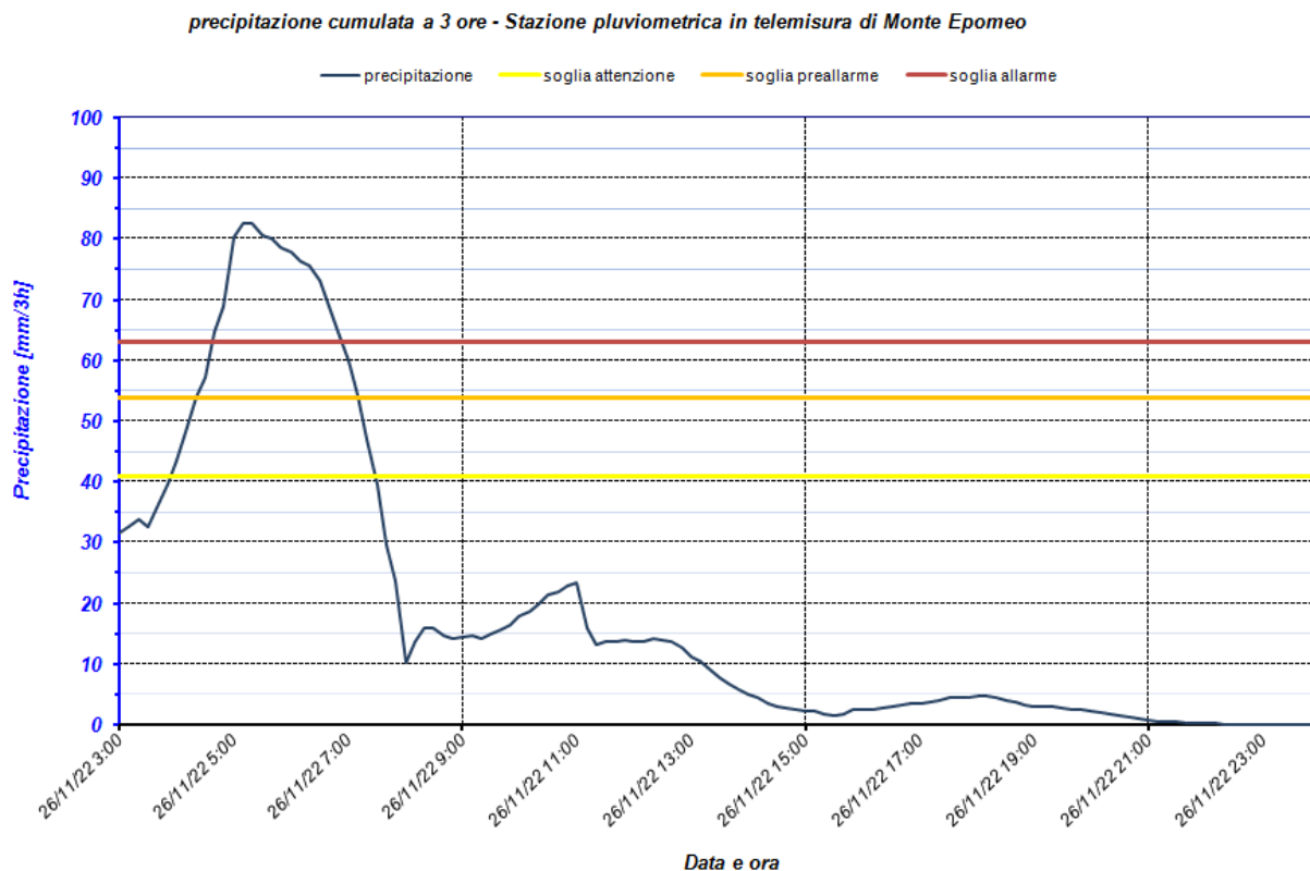
Figura 30. Stazione di Monte Epomeo: andamento temporale del precursore pluviometrico di durata 3 ore.
