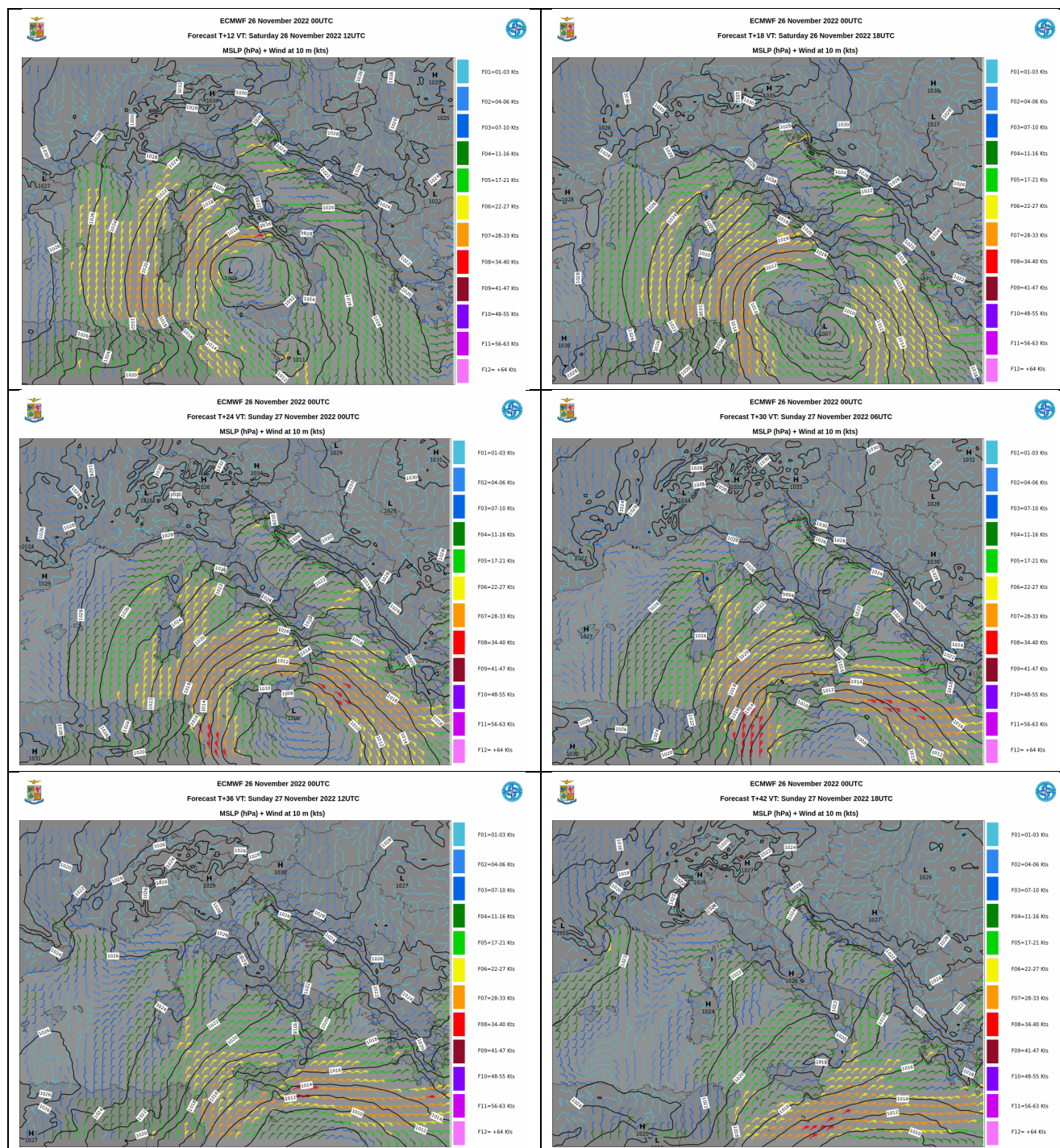
Figure 14 - Mappe di previsione della pressione media a livello del mare e del vento a 10m con step esarorio dalle ore 12UTC del 26 novembre 2022 alle 18UTC del 27 novembre 2022 del modello ECMWF (RUN delle 00 UTC del 26 novembre 2022).
