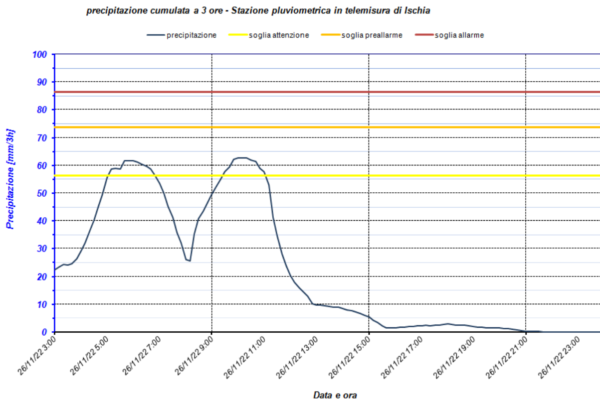
Figura 26. Stazione di Ischia: andamento temporale del precursore pluviometrico di durata 3 ore.
