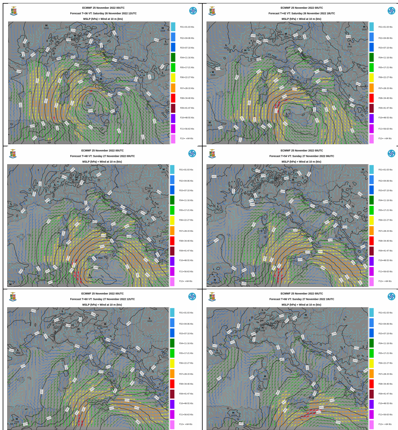
Figure 13 - Mappe di previsione della pressione media a livello del mare e del vento a 10m con step esarario dalle ore 12UTC del 26 novembre 2022 alle 18UTC del 27 novembre 2022 del modello ECMWF (RUN delle 00 UTC del 25 novembre 2022).
