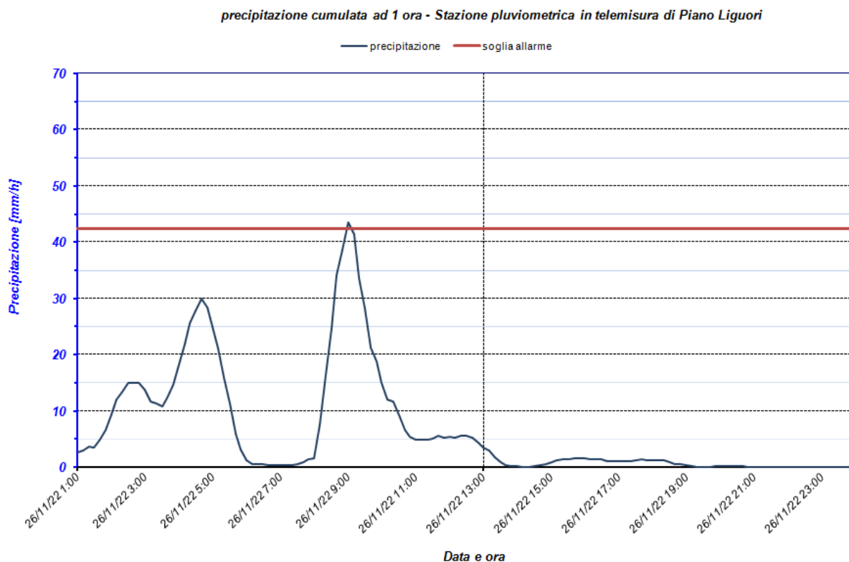
Figura 27. Stazione di Piano Liguori: andamento temporale del precursore pluviometrico di durata 1 ora.
