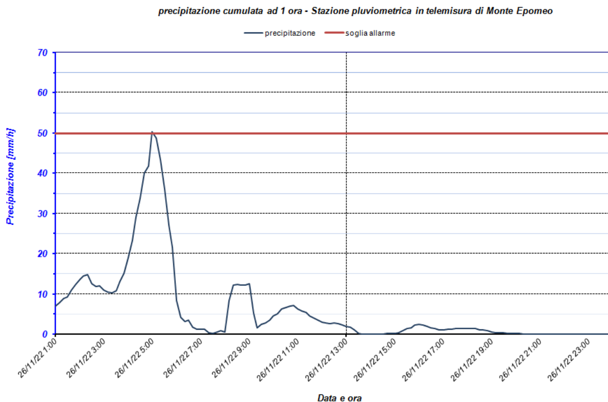
Figura 29. Stazione di Monte Epomeo: andamento temporale del precursore pluviometrico di durata 1 ora.
